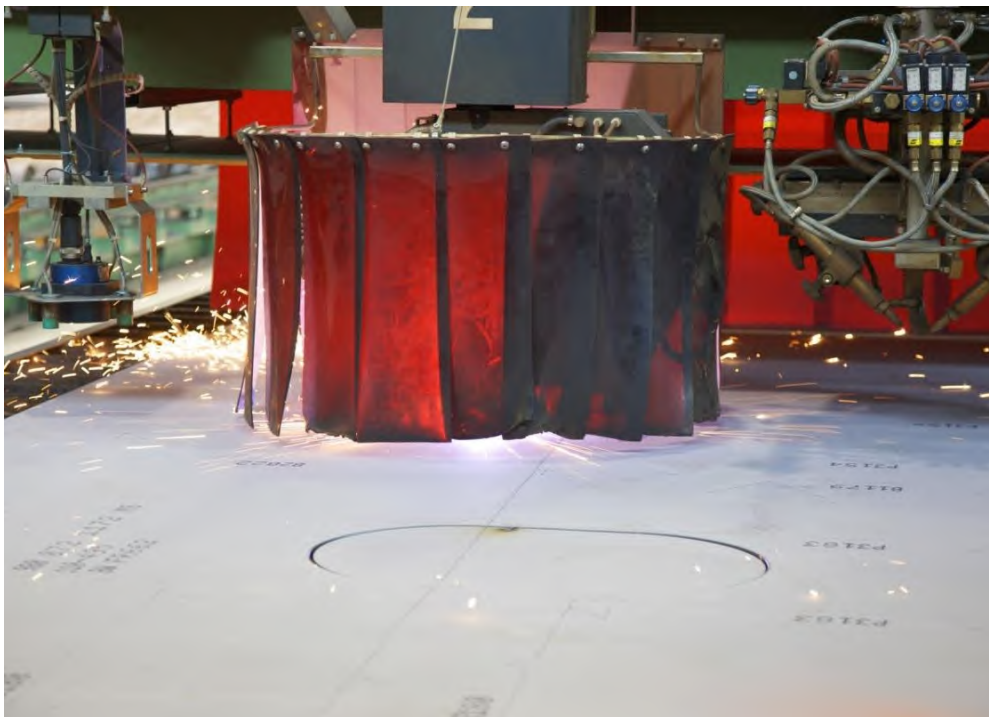
Abbildung 6 Brennbeginn der 1. Bauteils
